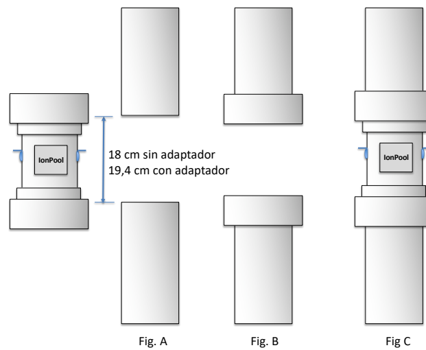
Figura 4 Instalación del electrodo
